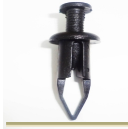
3852 KLİPS DAVLUMBAZ ,(90467-09093) TOYOTA Z0111
