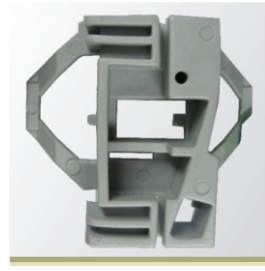
3959 KLİPS CAM MEKANİZMA L ARKA (4) POLO KLASİK VW
