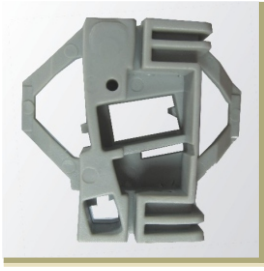
3957 KLİPS CAM MEKANİZMA(6) ÖN VW, POLO KLASİK R
